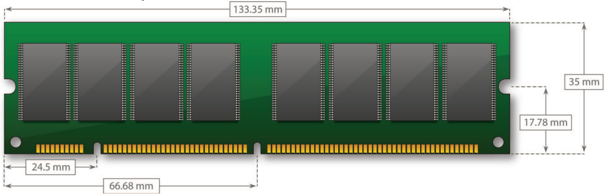
DDR DIMM (184 pin)
